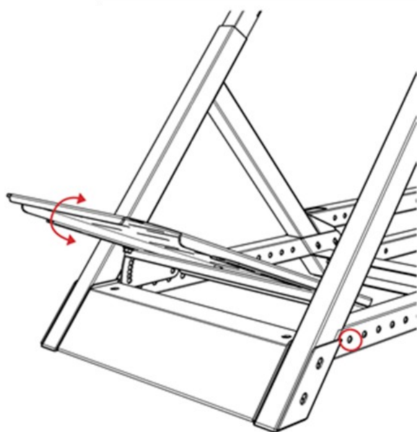
NASTAVENÍ ÚHLU A DÉLKY DESKY PEDÁLU
