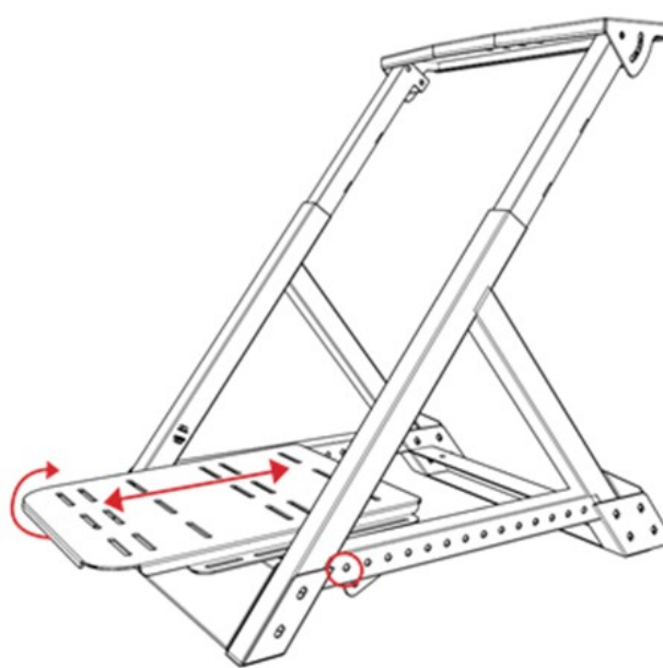
NASTAVENÍ ÚHLU A DÉLKY DESKY PEDÁLU
