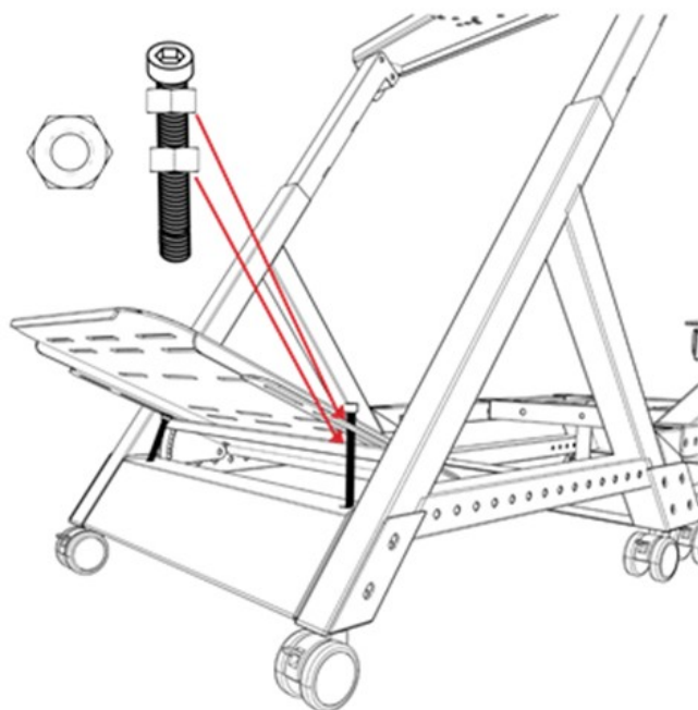
ŠROUB PRO UPEVNĚNÍ PEDÁLU
